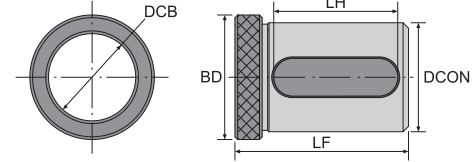
寸法 Dimension(mm)
