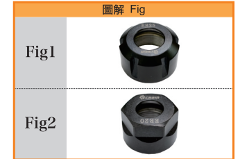
寸法 Dimension(mm)
