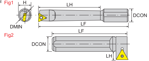
寸法 Dimension(mm)
