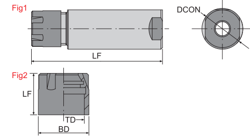
寸法 Dimension(mm)
