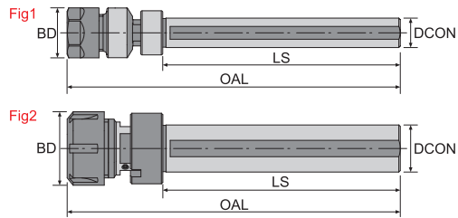
寸法 Dimension(mm)
