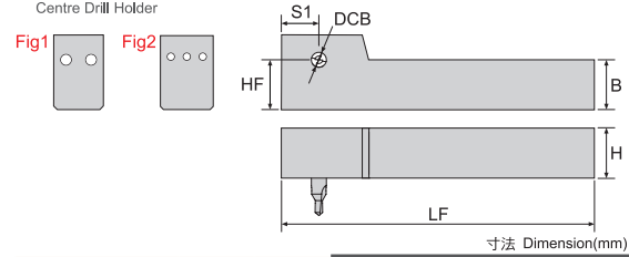
寸法 Dimension(mm)
